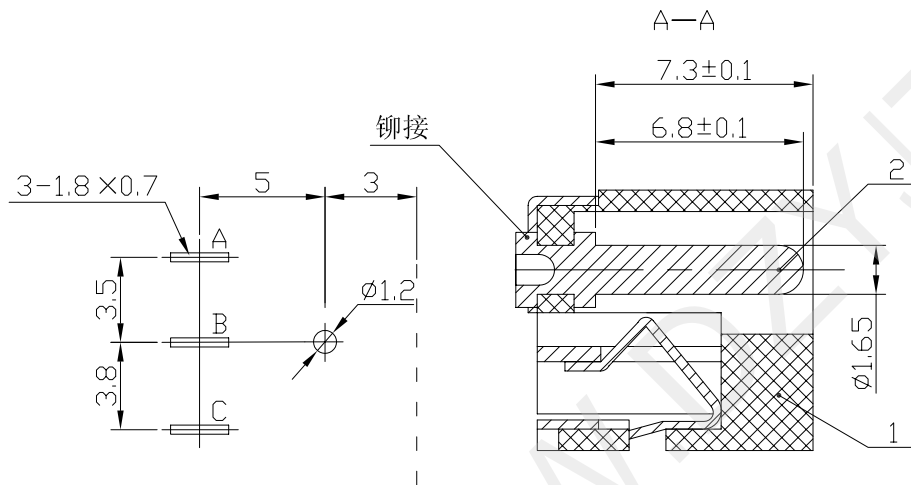
安装尺寸图
